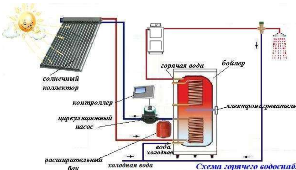
Схема горячего водоснабжения и отопления с применением солнечного коллектора
