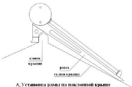
А. Установка рамы на наклонной крыше
