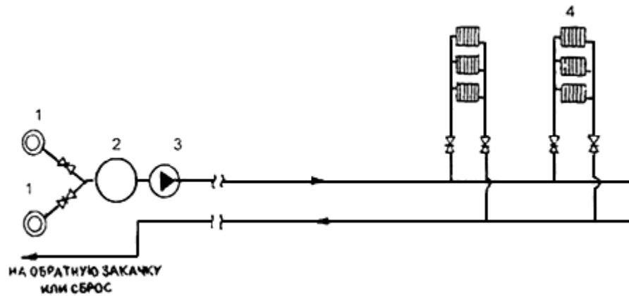
1 - геотермальные скважины; 2 - промежуточный бак-аккумулятор; 3 - сетевой насос; 4 - отопительные приборы Рисунок Д4.4 - Геотермальная система теплоснабжения с зависимым присоединением отопления (ГВ отсутствует)
