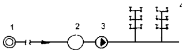
1 - геотермальная скважина; 2 - бак-аккумулятор; 3 - сетевой насос; 4 - водоразборный кран ГВ Рисунок Д4.5 - Открытая однотрубная геотермальная система горячего водоснабжения
