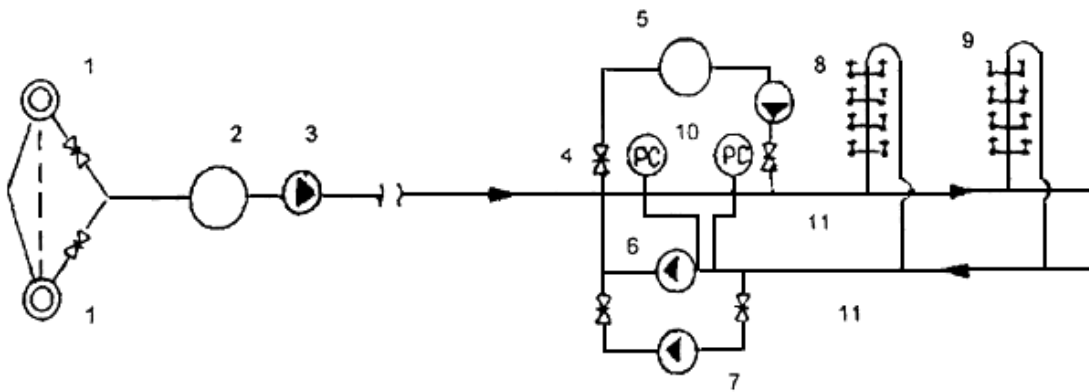
1 - геотермальные скважины термоводозабора; 2 - сборный бак-аккумулятор геотермальной воды; 3 - сетевой насос; 4 - регулятор слива; 5 - бак-аккумулятор распределительной сети; 6, 7, 8 – сетевой циркуляционный и подпиточный насосы распределительной сети; 9 - водоразборный кран; 10 - регулятор подпитки; 11 - двухтрубная распределительная сеть Рисунок Д4.6 - Открытая однотрубная геотермальная система горячего водоснабжения с двухтрубной распределительной сетью
